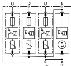
Schéma de principe du circuit DG M TT CI 275
