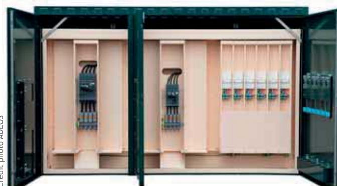
Vue côté branchements forains
