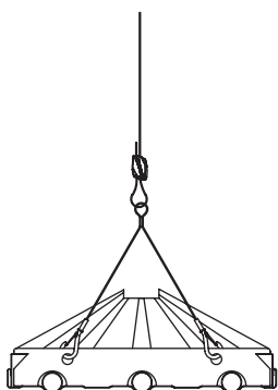
Accessoire Y embout crochet sur un panneau radiant
