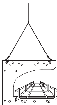
Accessoire Y avec étrier G sur un chemin de câble
