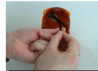
Insérer les gaines fournies
