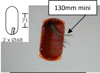
Percer et fixer la boîte
