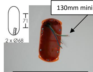
Percer et fixer la boîte
