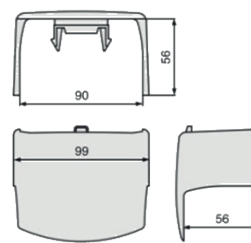
NTAC Té de dérivation TA-C
